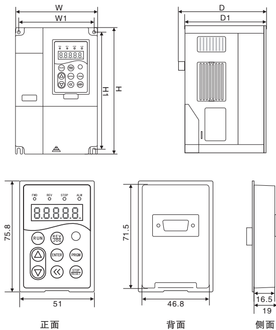
0.4-2.2KW系列机箱规格表
