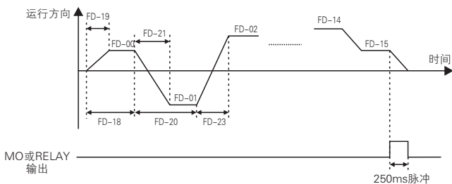
简易PLC示意图
