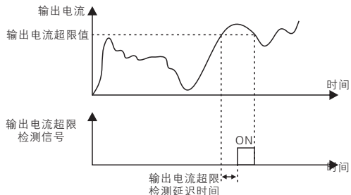
输出电流超限检测示意图
