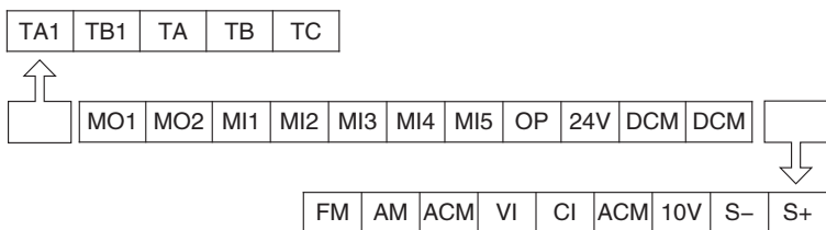
11kw(含11kw)以上控制回路接线端子图
