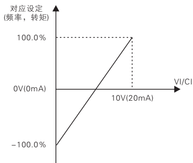
模拟给定与设定量的对应关系
