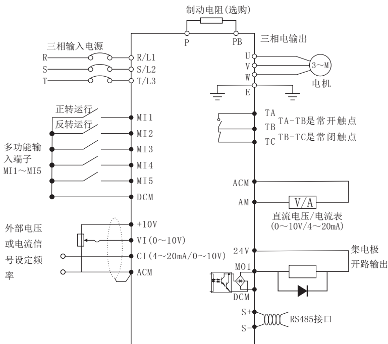
2.2kw及以下标准配线图
