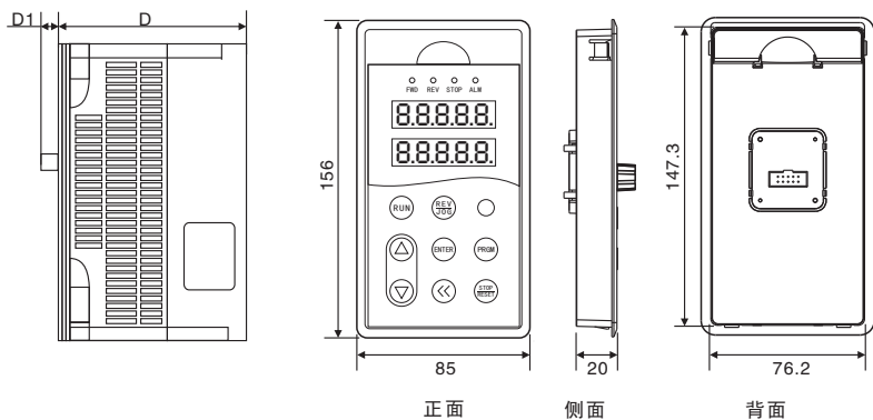
键盘托尺寸图
