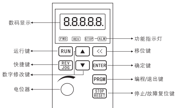
单显示操作面板示意图
