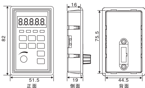
0.4-2.2KW系列机箱规格表
