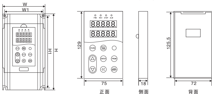
键盘尺寸图
