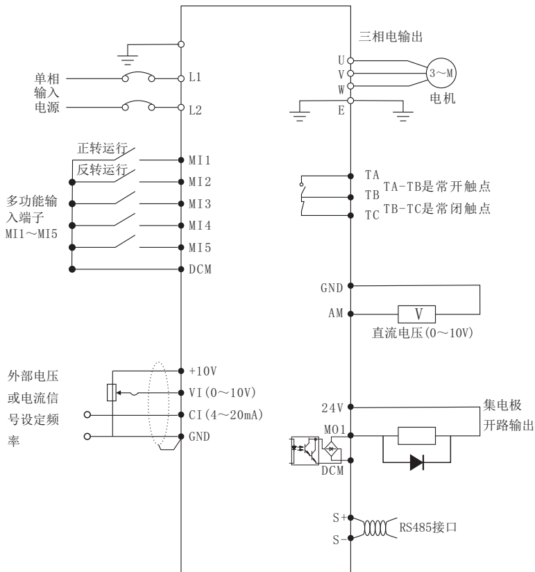
M型0.4~1.5kw标准配线图
