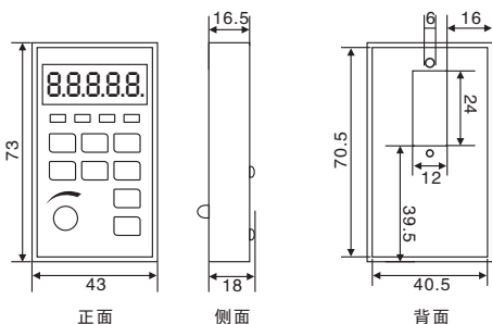
键盘尺寸图
